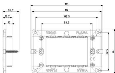
Vista ingombri
